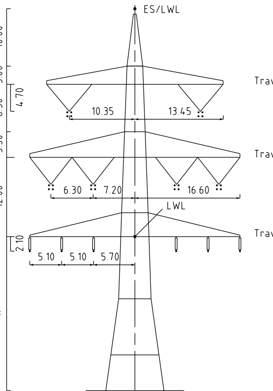
Mast Nr. 169
