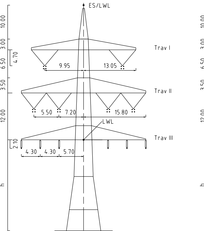
Mast Nr. 167-168, 170
